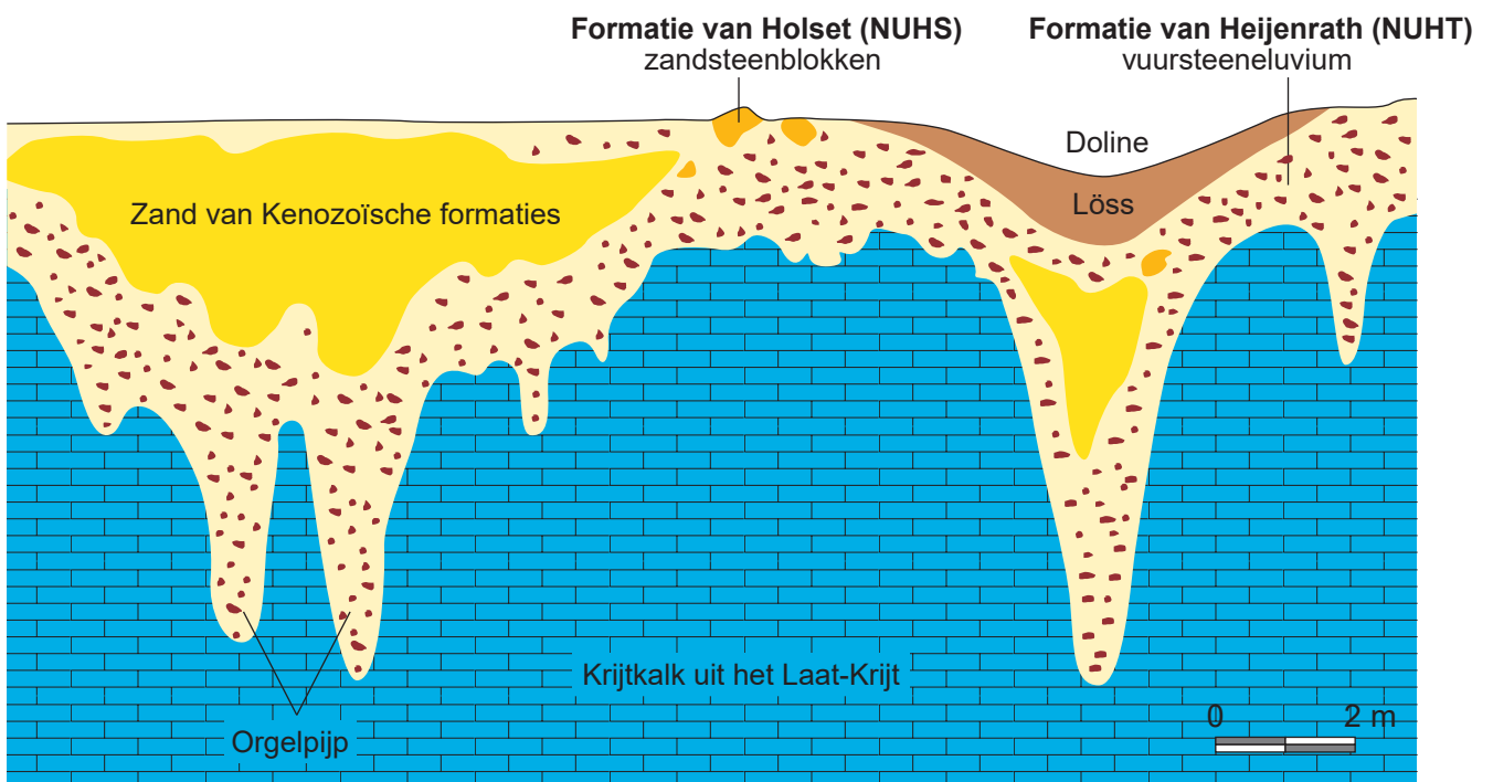
Schematische doorsnede bij het Vylenerbos (Zuid-Limburg) met de stratigrafische posities van de formaties van Holset en Heijenrath.
