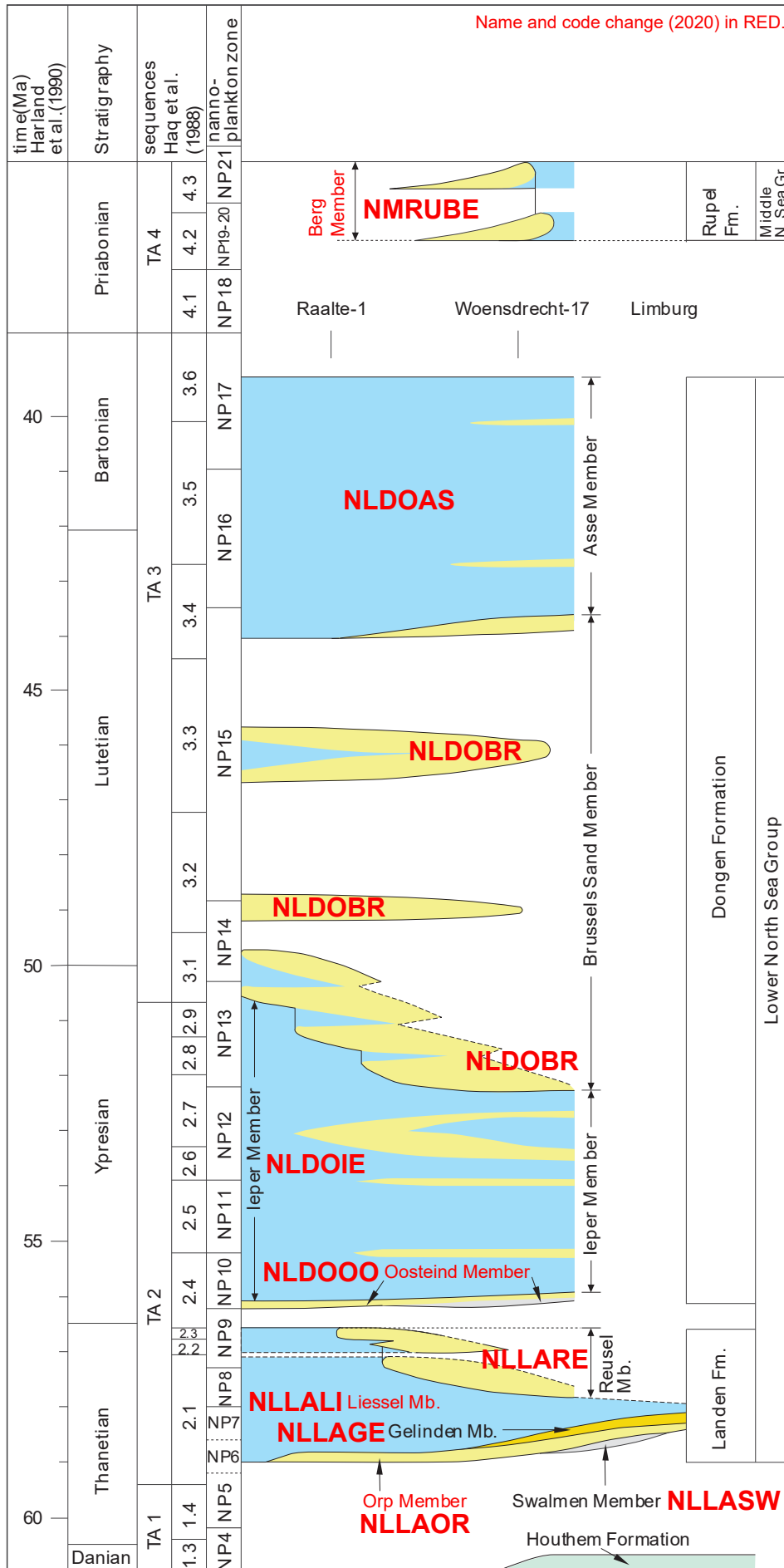
Modified after: Van Adrichem Boogaert & Kouwe (1997). Stratigraphic nomenclature: Section I - Tertiary - Mededelingen Rijks Geologische Dienst 50
