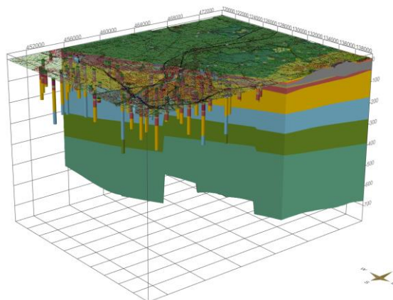
Figuur 9: Voorbeeld van een snijvlak door een lagenmodel waarbij de boringen zichtbaar blijven.
